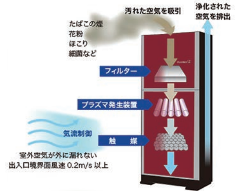
喫煙室用プラズマ脱臭機
